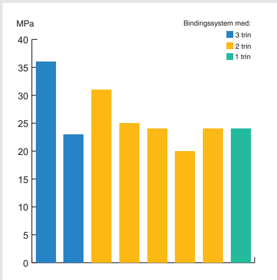
Fig. 1. Binding af plast til emalje formidlet af en række tretrins-, tottrins- og éttrinsbindingssystemer.
